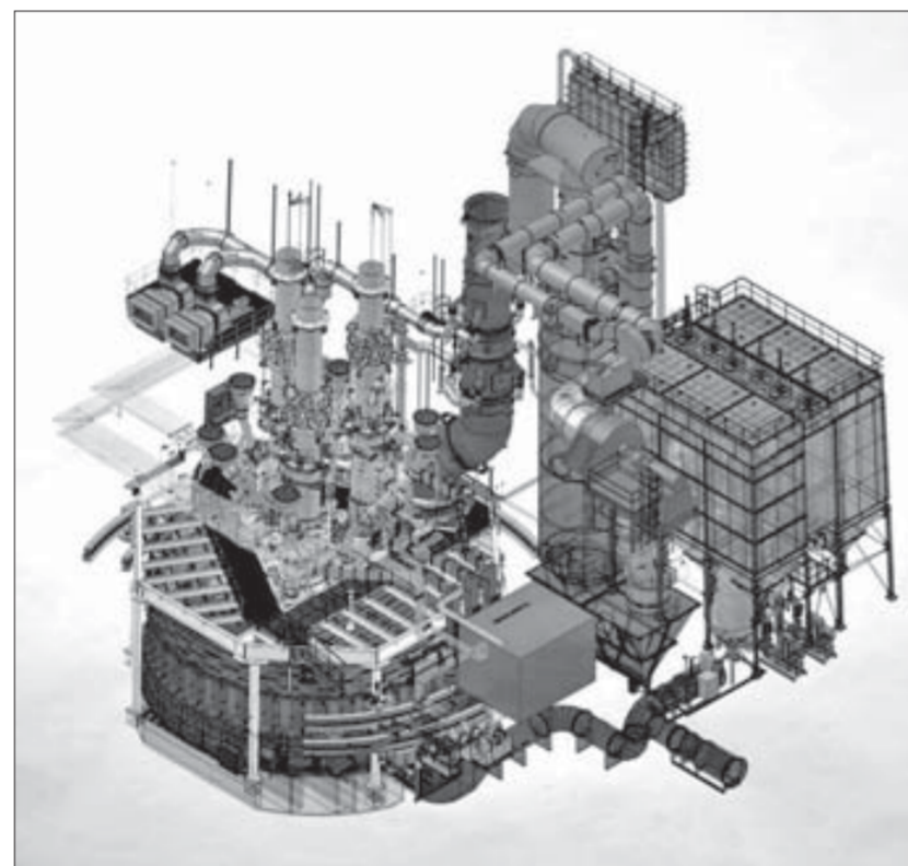
Изометрическая схема ОЭП-4
