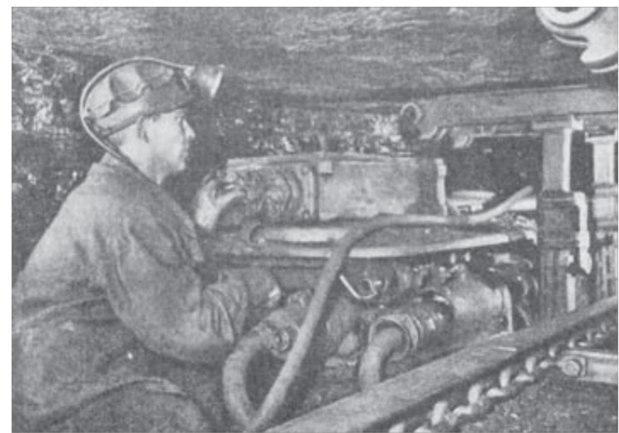
Врубовая машина
